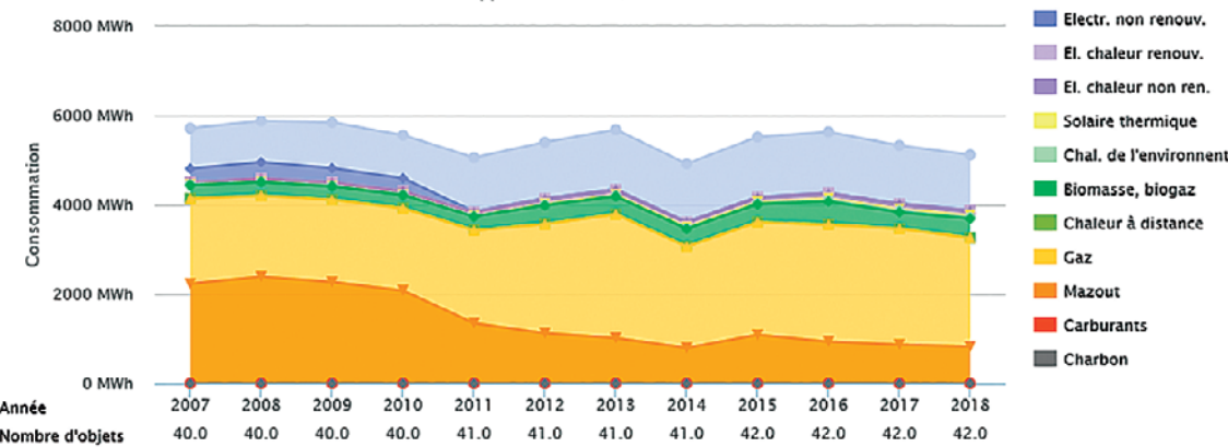
Evolution de la consommation d'énergie Rapport du 01.01.2007 au 31.12.2018
