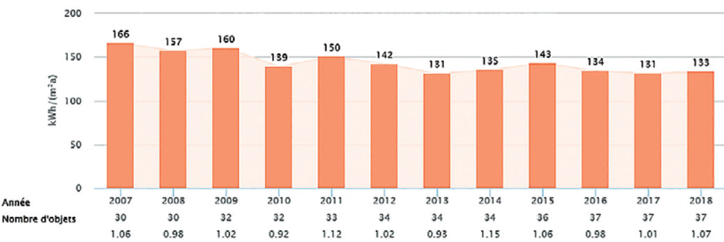
Evolution des indices énergétiques: Chaleur Rapport du 01.01.2007 au 31.12.2018
