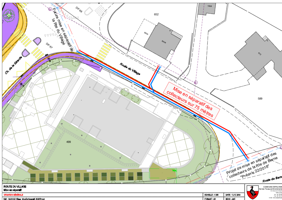
Figure 4 : Plan des travaux sur la Route du Village
