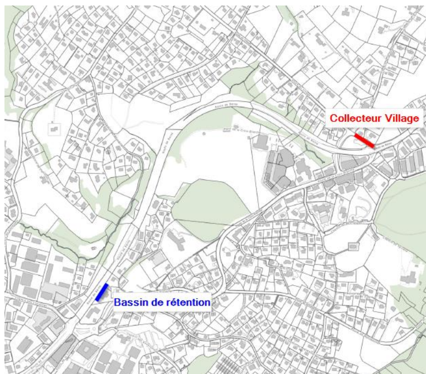
Figure 1 : Plan de situation avec l'ouvrage et les collecteurs faisant l'objet du présent préavis
