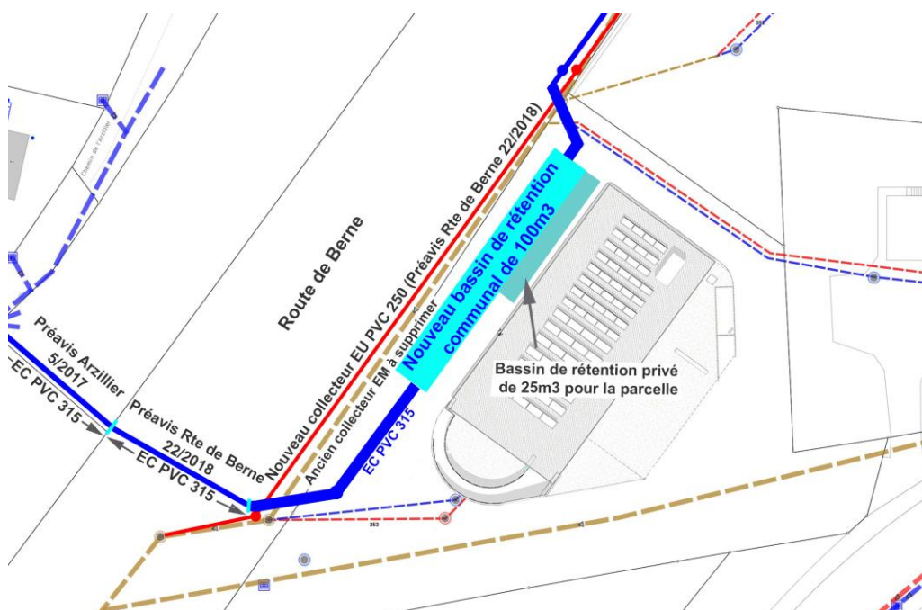
Figure 3 : Plan des travaux pour le bassin de rétention du quartier des Geais
