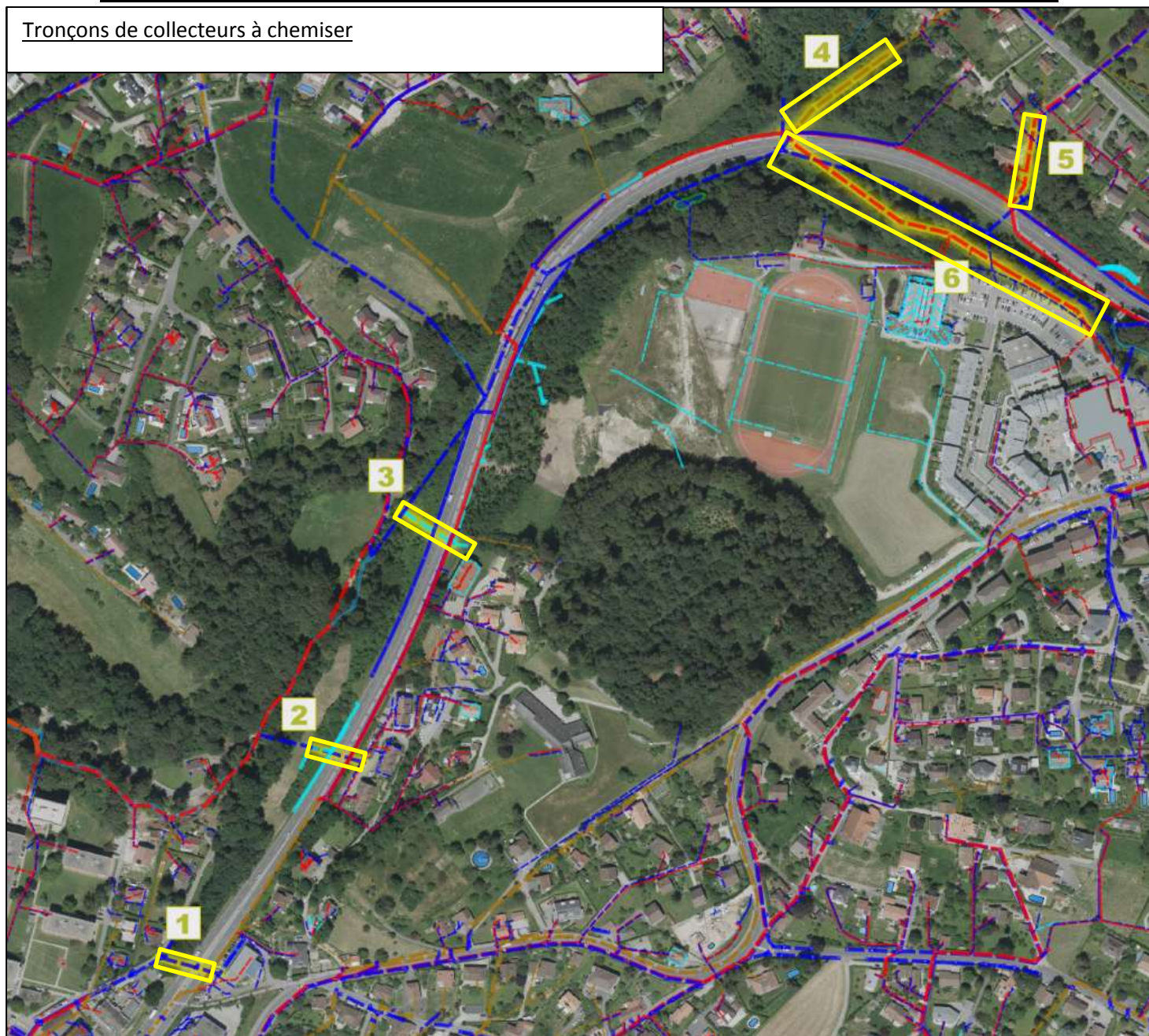
Figure 1 : Plan de situation avec les tronçons de collecteurs faisant l'objet du présent préavis
