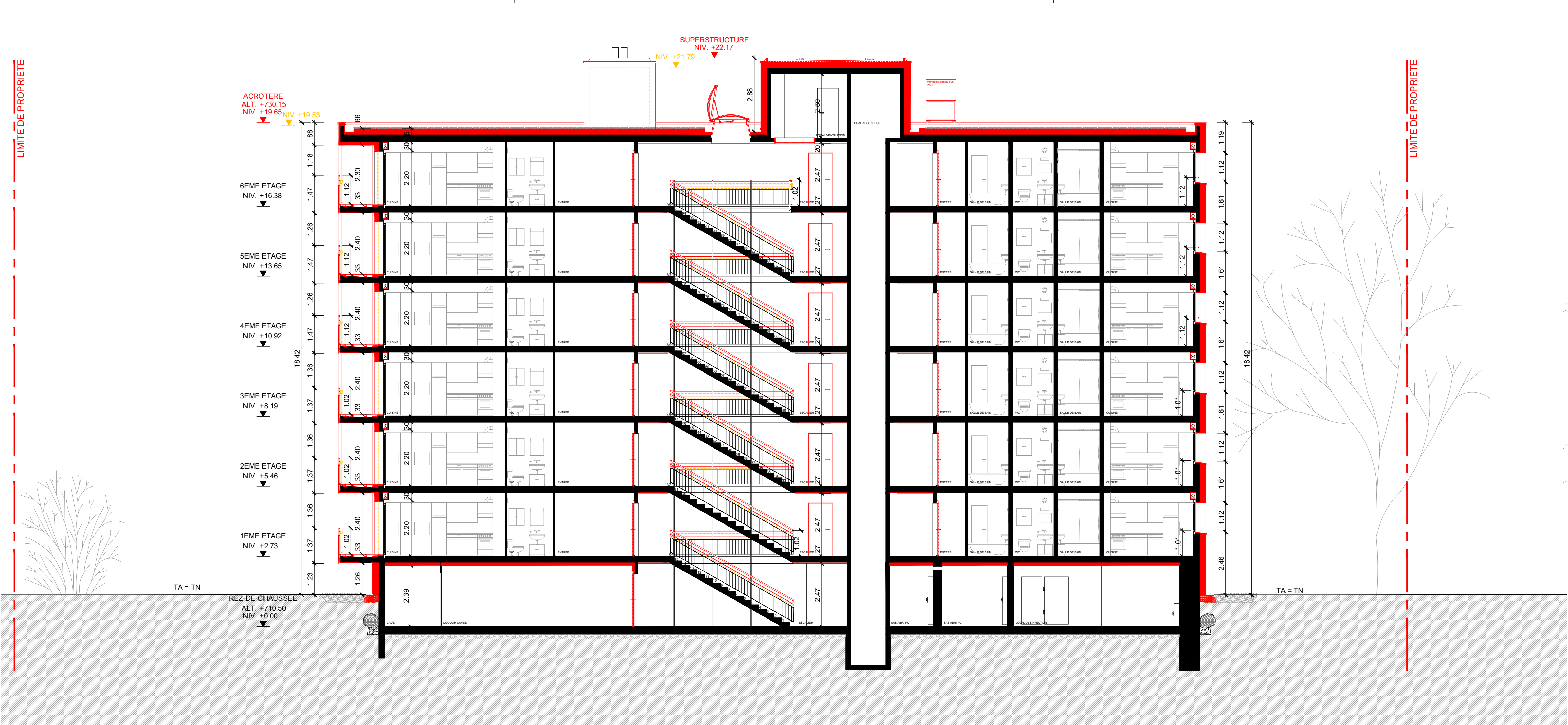
COUPE A-A
