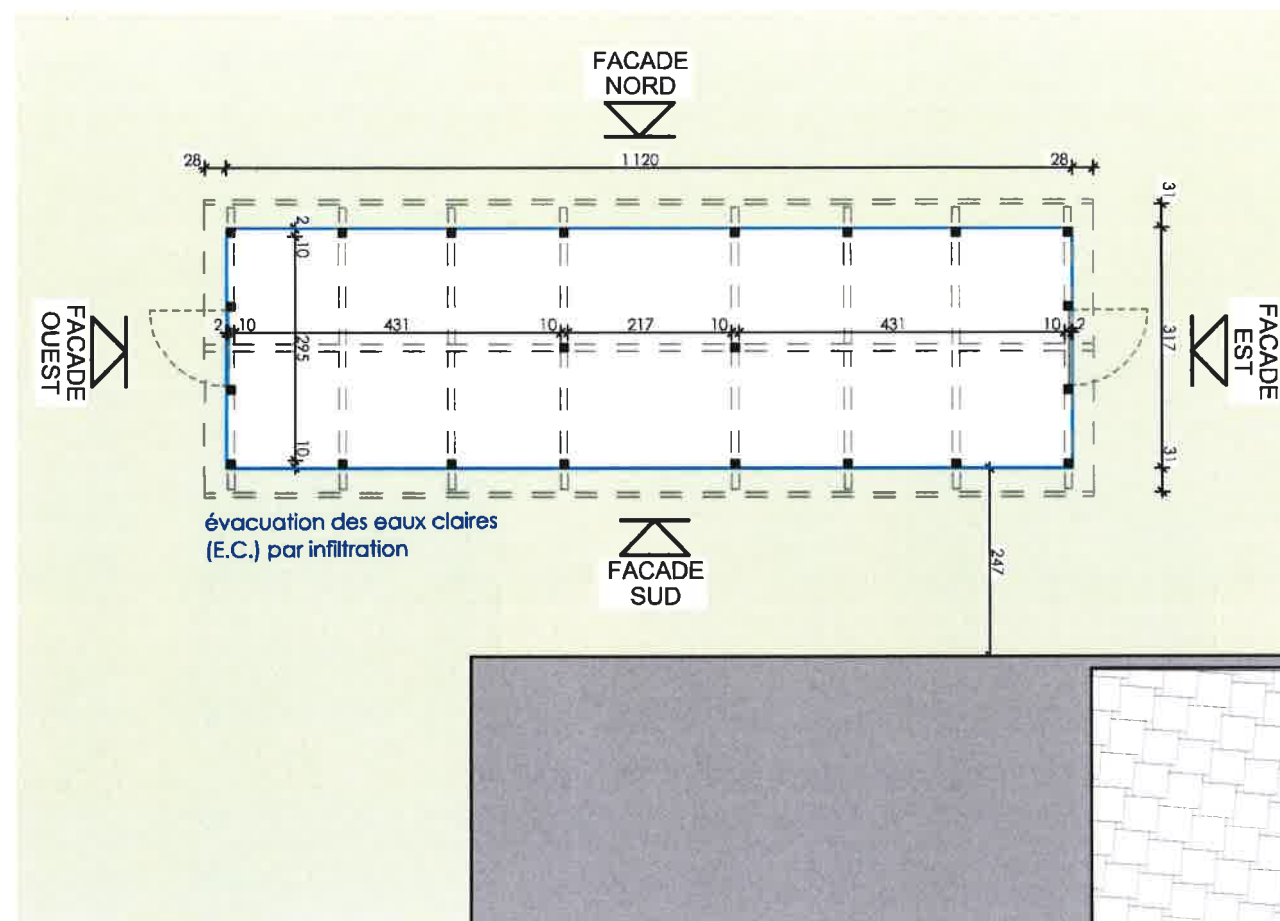
Rez-de-chaussée
