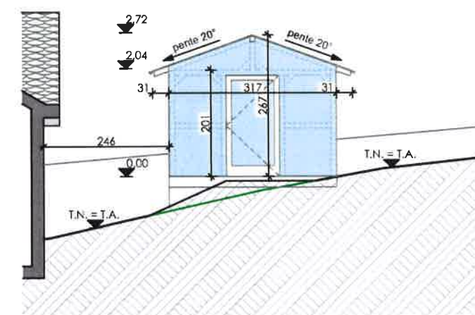
Façade Est
