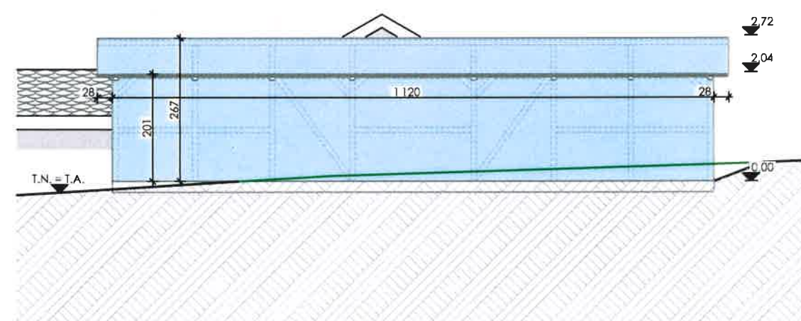
Façade Nord
