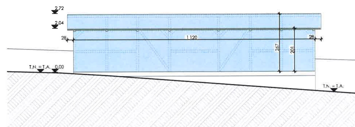
Façade Sud
