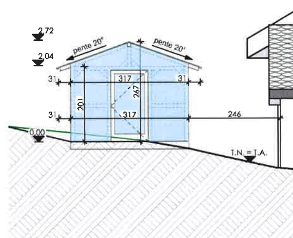
Façade Ouest
