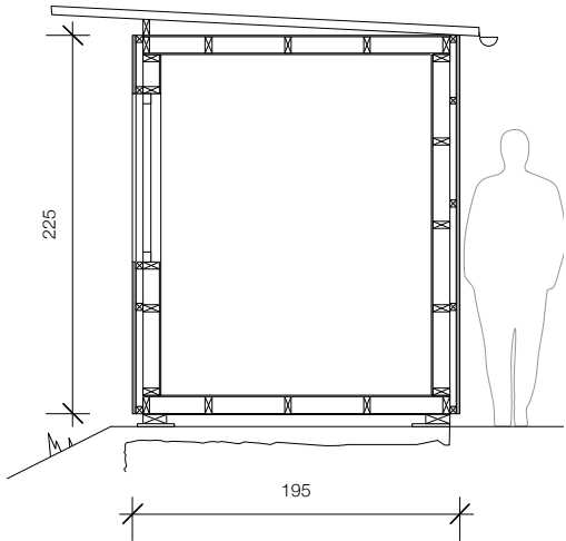
coupe 1 :50
