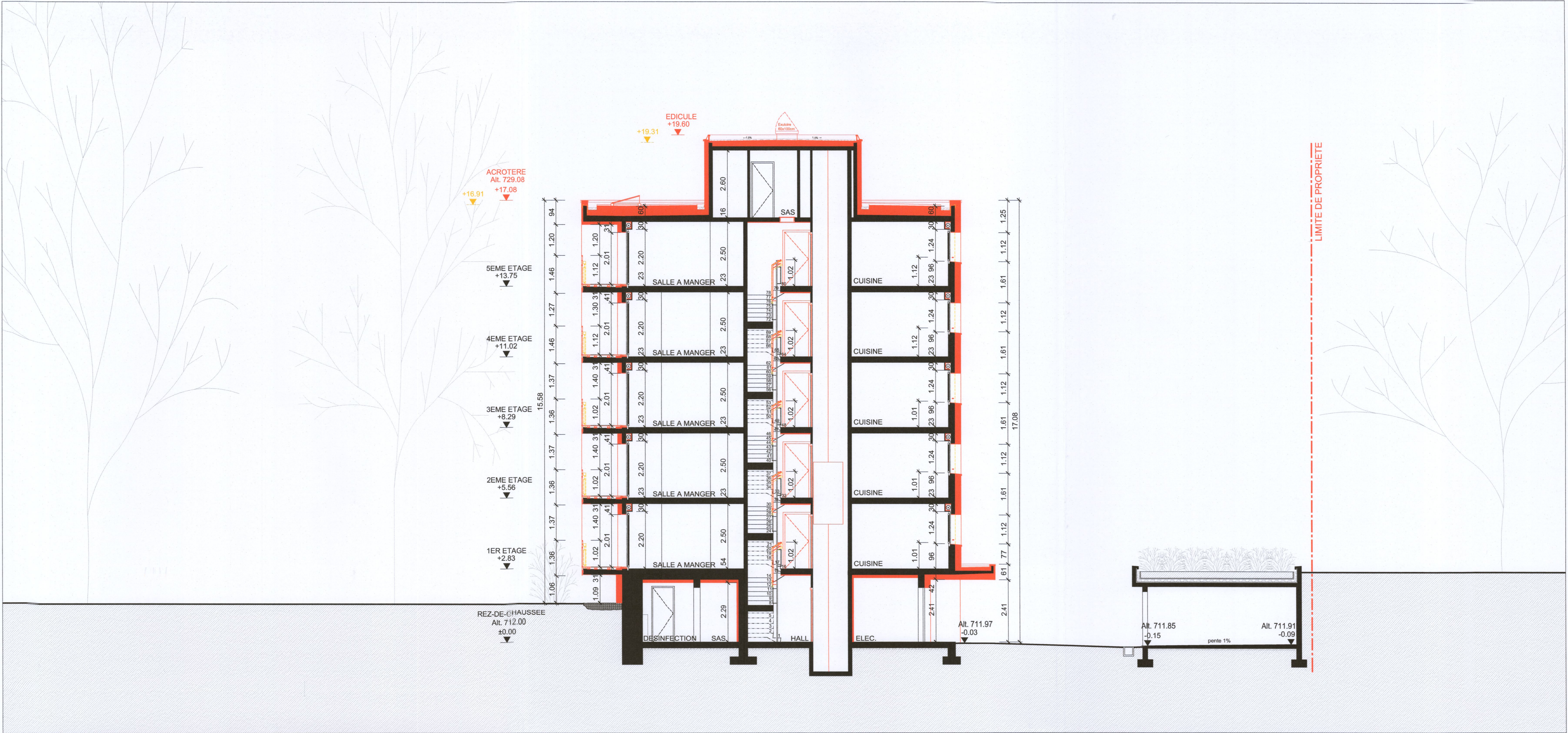
COUPE A-A
