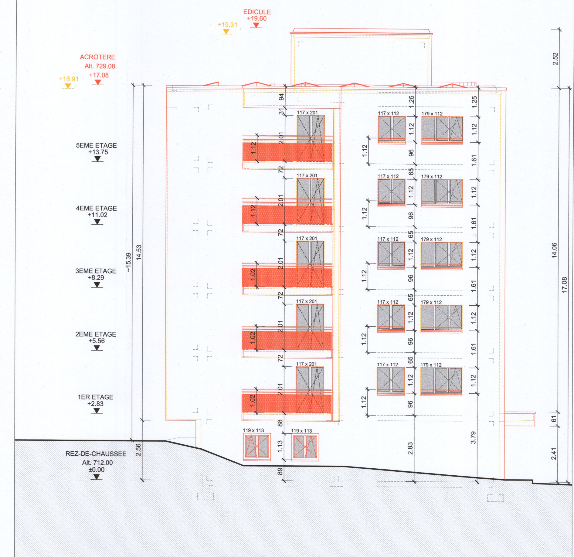
FACADE EST
