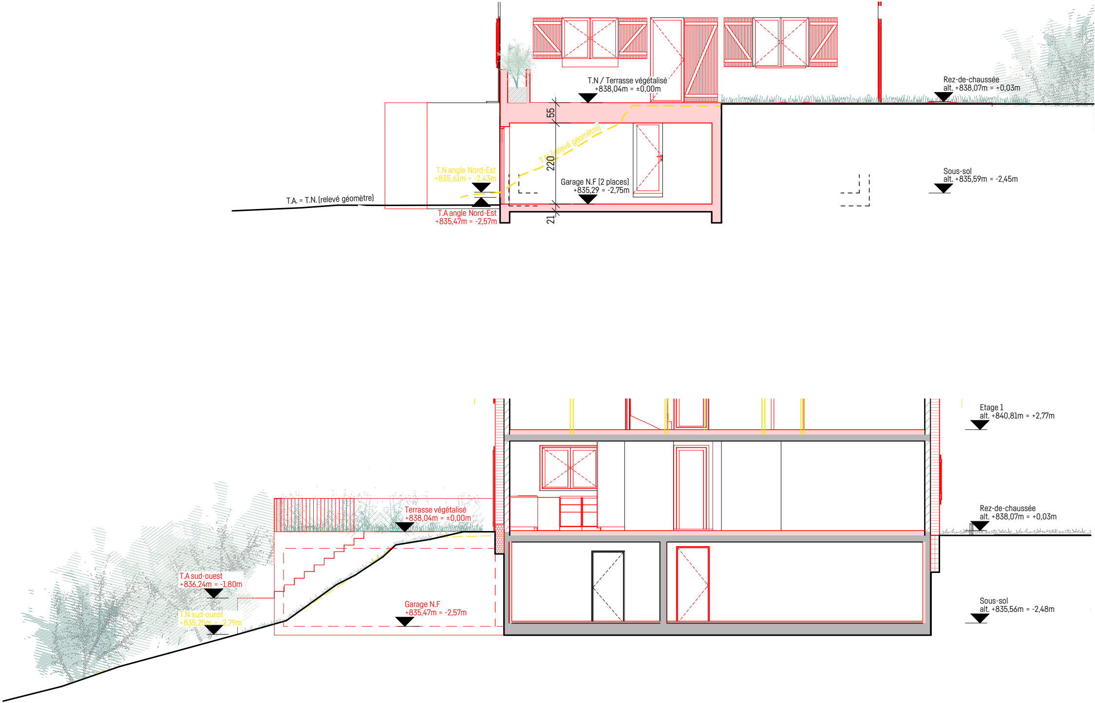
FAÇADE GARAGE - SUD
